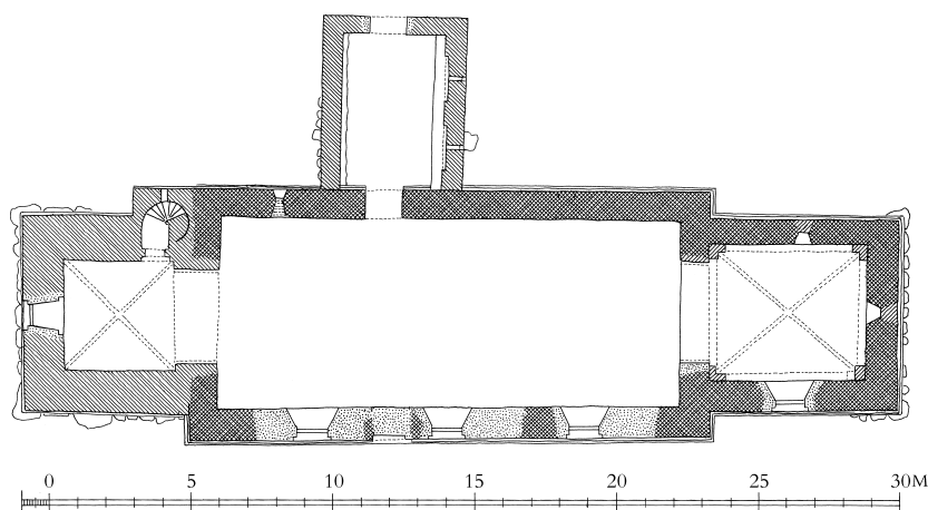
Fig. 6. Plan 1:300. Målt af Sven Fritz 1941, suppleret af Peter Duun 2009 samt suppleret og tegnet af Hugo Johannsen 2010. – Grundriss.
