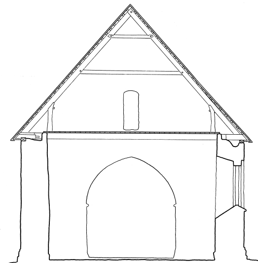
Fig. 5. Tværsnit gennem skibet set mod øst. 1:150. Målt og tegnet af Peter Duun 1999 og 2010. – Querschnitt durch Schiff gegen Ost.
