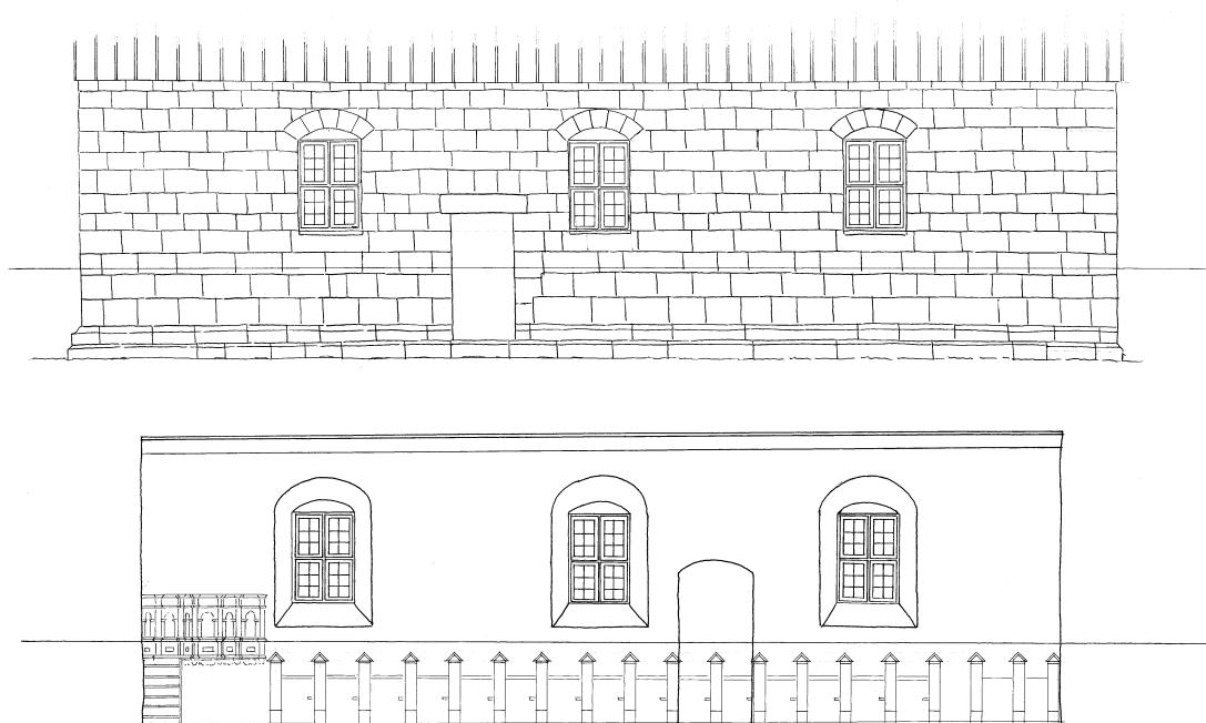
Fig. 10a-b. Forslag til ændring af skibets sydside, jf. fig. 8. 1:150. a. Ydre. b. Indre. Tegnet af Sven Fritz 1941. – Vorschlag zur Änderung der Südseite des Schiffes.
