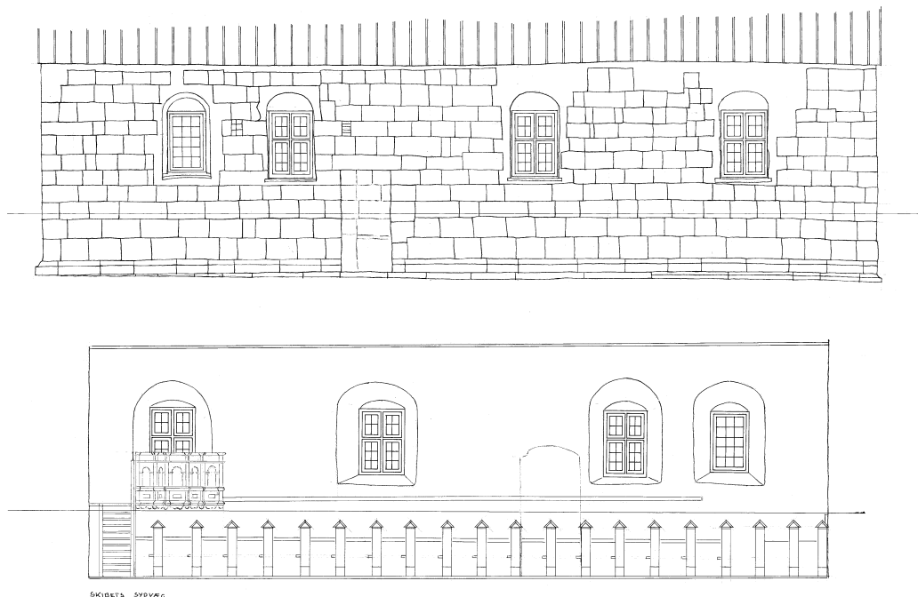
Fig. 8a-b. Opstalter af skibets sydside. 1:150. a. Ydre. b. Indre. Målt og tegnet af Sven Fritz 1941. – Aufrisse der Südseite des Schiffes.
