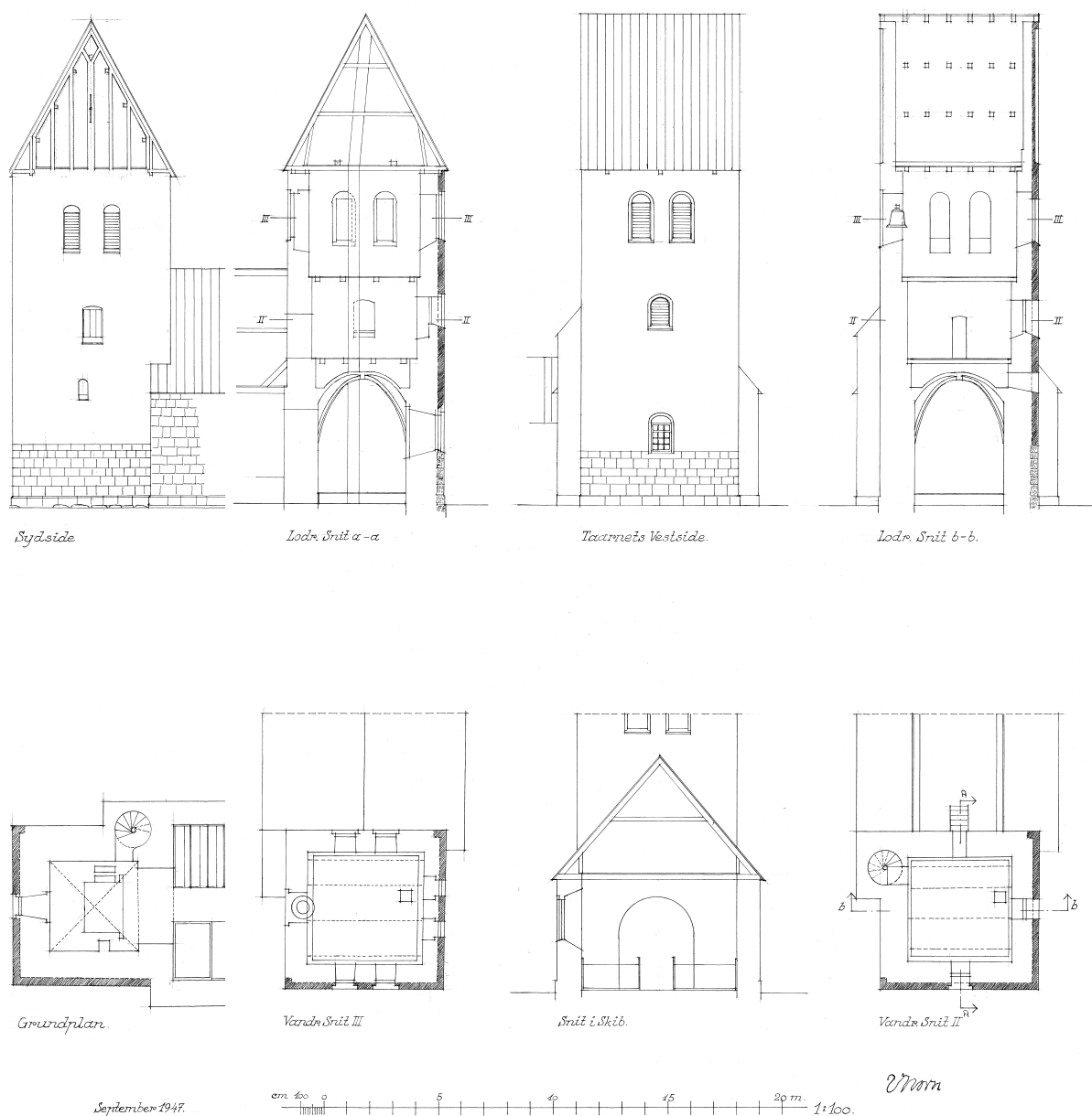
Fig. 14. Planer, snit og facader med forslag til tårnets restaurering, 1:300. Viggo Norn 1947. Horsens Museum. – Grundrisse, Schnitte und Fassaden mit Vorschlag zur Restaurierung des Turmes.
